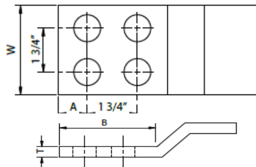
OFFSET LUG
