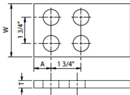
STRAIGHT LUG
